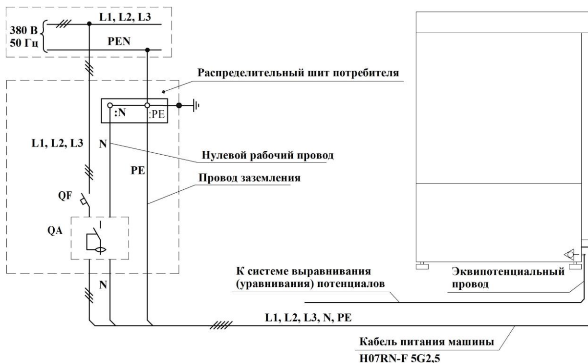
Рисунок 7 – Схема подключения к электрической сети
